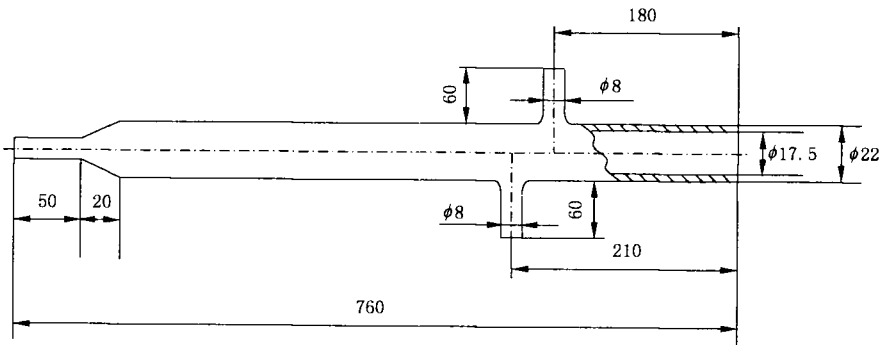
图 2 石英管
